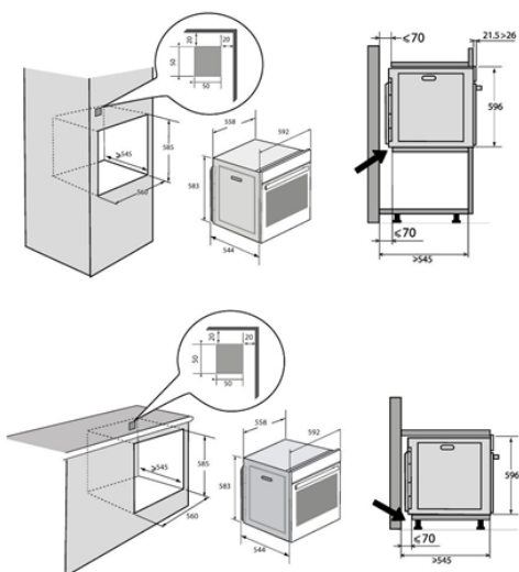
Schéma pro vestavbu BOP75xx, BOH75xx
